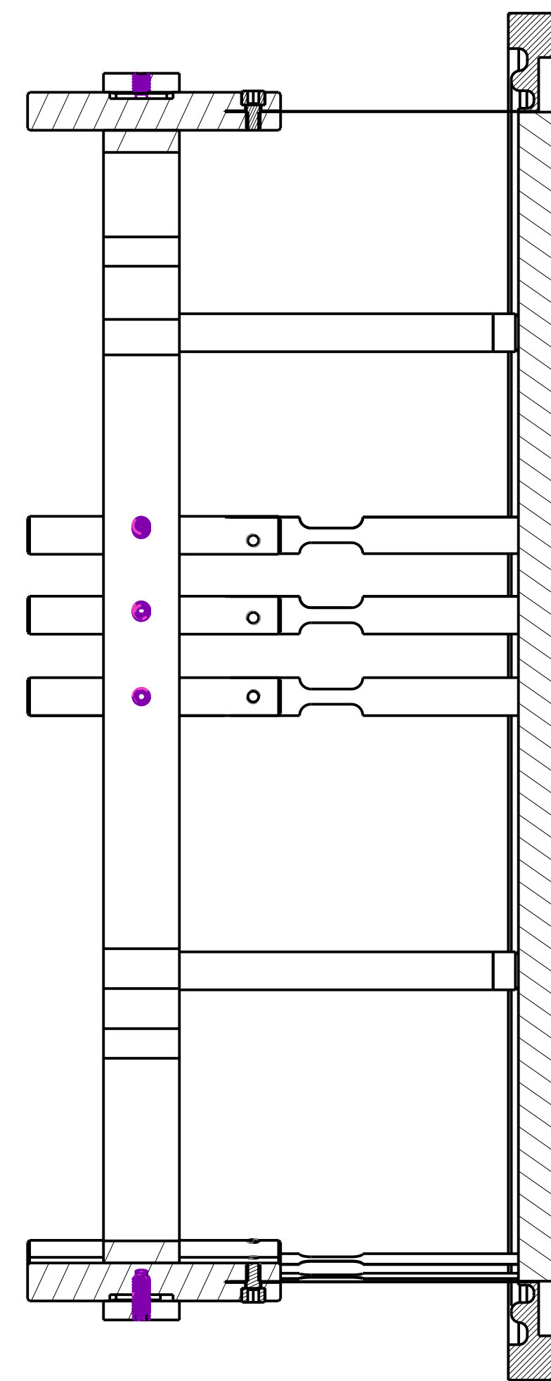
SECTION A-A
